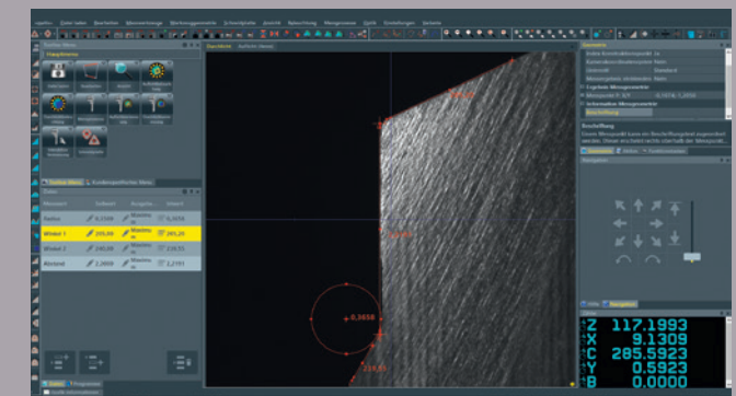
Werkzeuganalyse »metis« – vermisst und dokumentiert beliebige Konturen, Radien, Winkel, Abstände und Defekte (Verschleiß) im Auflicht.
